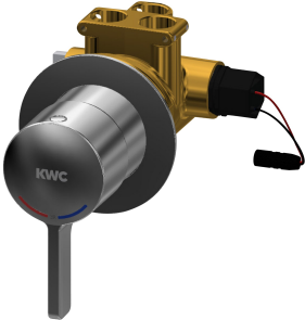
Funktionsblock
