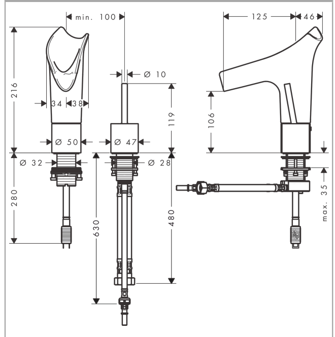
Maßzeichnung
