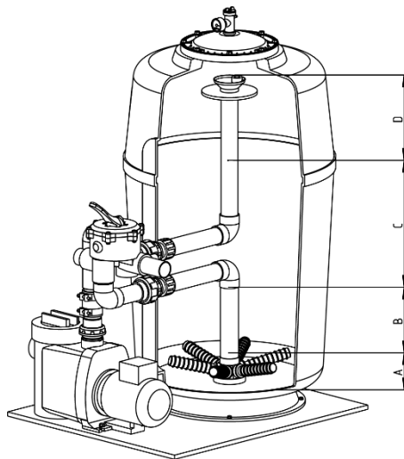
Abb. D-3: Schüttschema zum GENO-mat F 600 H
