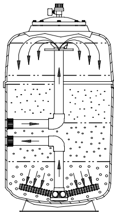
Abb. B-2: Filtration GENO-mat F 600
