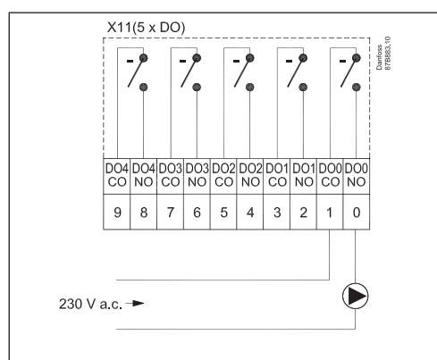
Beispiel 2: 230 V AC, Steuerung einer Umwälzpumpe
