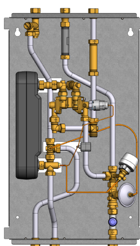
KW-Zufluss von oben mit KWZ-Paßstück.
