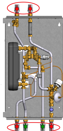
Akva Lux II Reno Eco mit Kugelhahn-Set 145H4015
