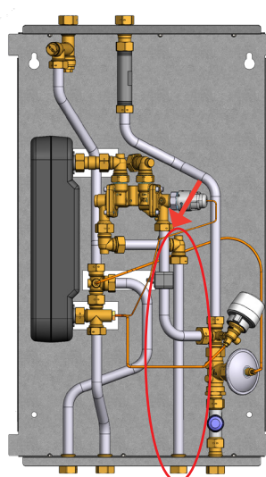
Akva Lux II Reno Eco Kaltwasseranschluss von unten.
