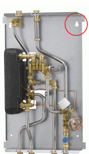
Akva Lux II Reno Eco ohne Rohrisolierung
