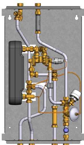
KW-Zufluss von unten mit KWZ-Paßstück.
