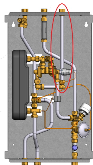
Akva Lux II Reno Eco Kaltwasseranschluss von oben.
