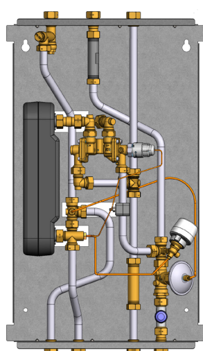
KW-Zufluss von unten mit KWZ-Paßstück. KW-Abfluss oben.
