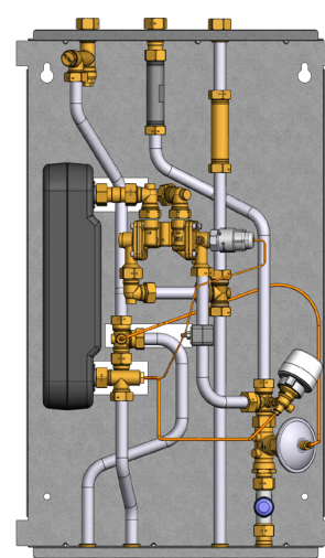
KW-Zufluss von oben mit KWZ-Paßstück und KW-Abfluss unten.
