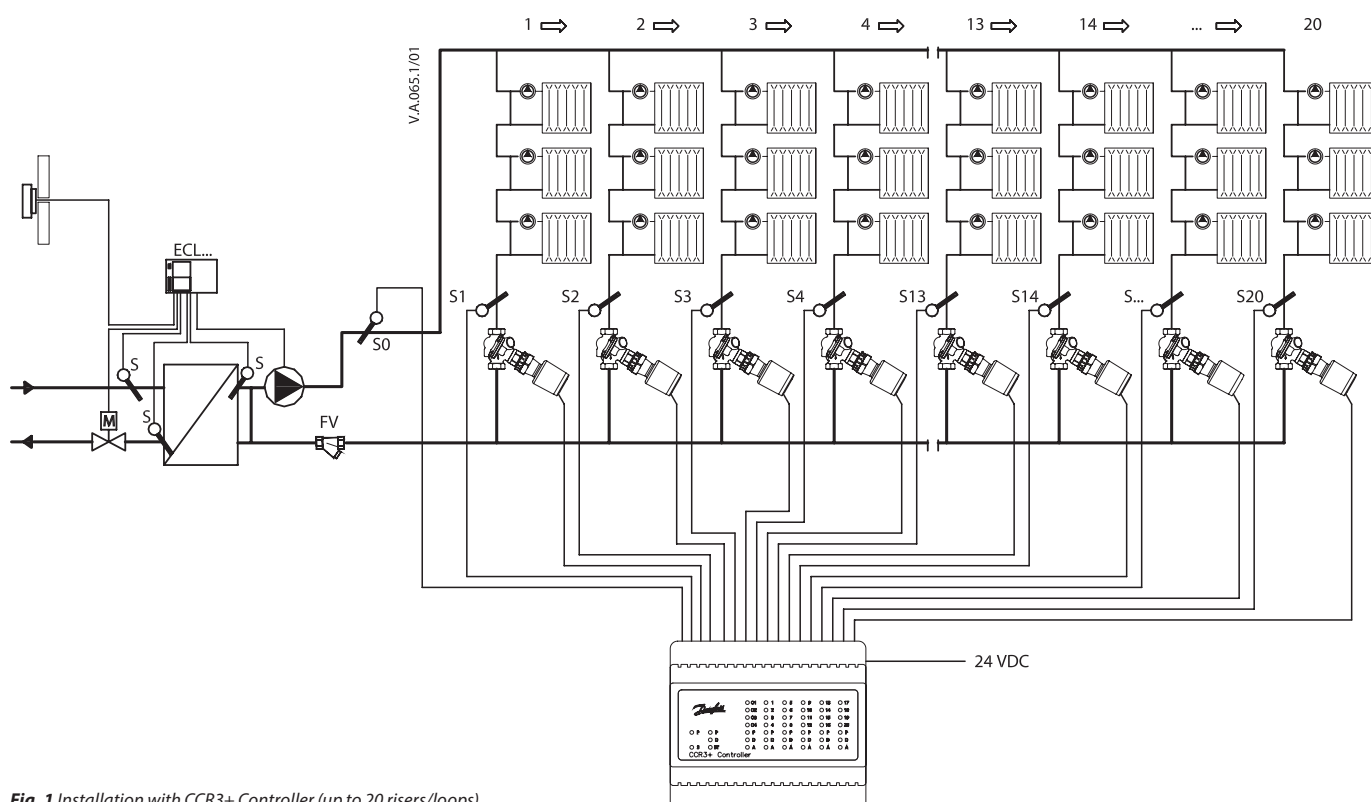
Abb. 1 Installation mit CCR3+ Regler (bis zu 20 Stränge/Kreise)
