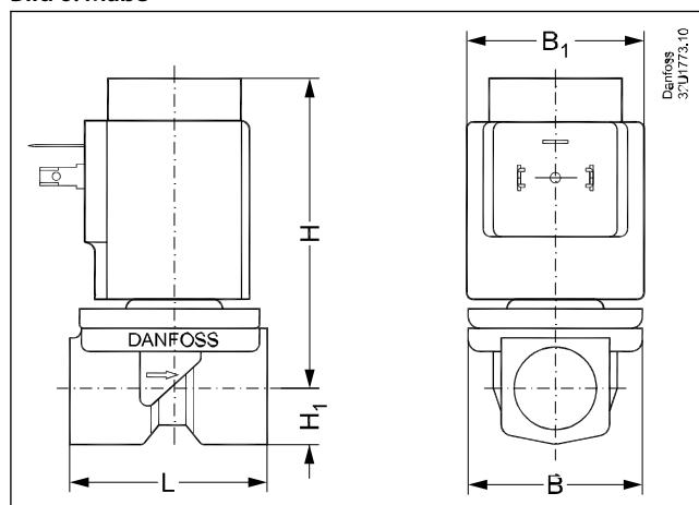
Bild 6: Maße
