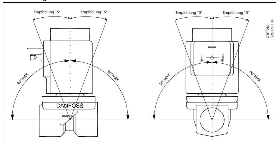
Bild 7: Montagewinkel
