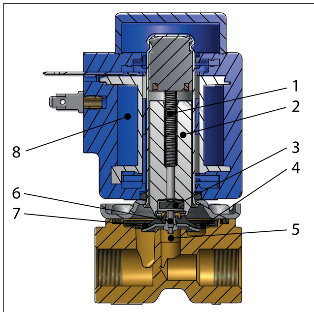
Bild 1: Funktion NC
