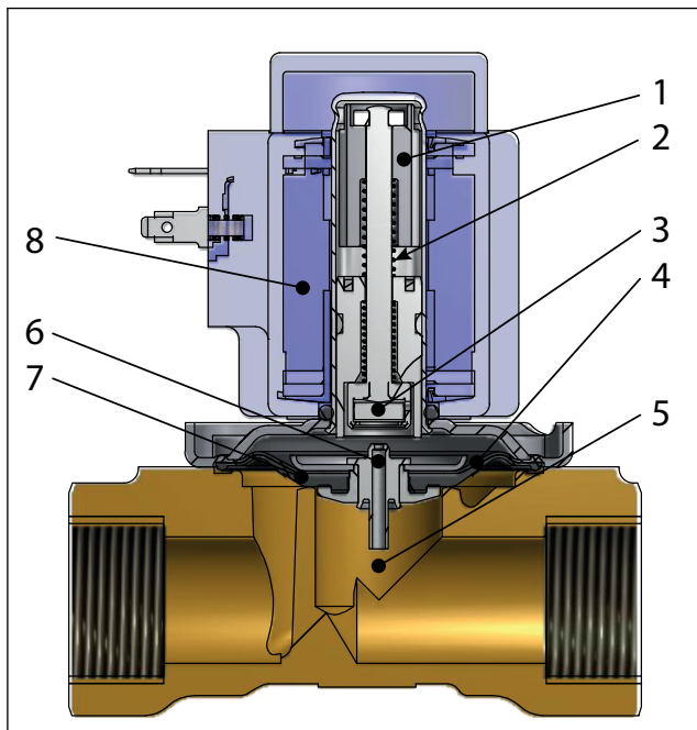
Bild 2: Funktion NO
