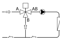
Abb. 1: Misch- oder Verteilanschluss
