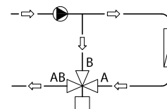
Abb. 3: Mischventil mit verteilender Wirkung
