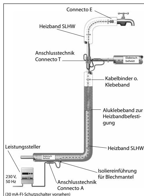
Montagebeispiel
